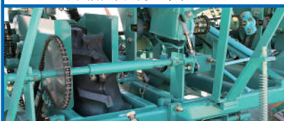
深耕爪取付金具 4畦
