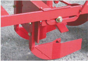
TDW用種子溝切り
