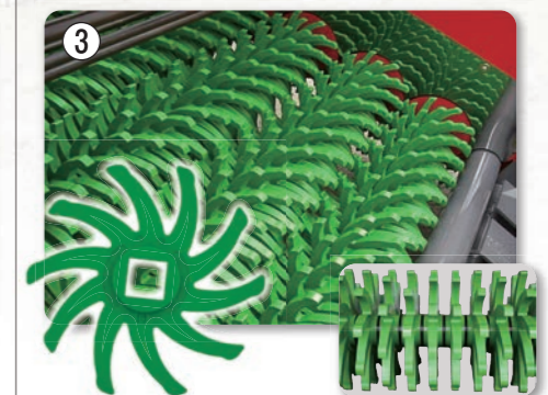
ウレタンゴム製のスターローラーは土塊を粉砕するとともに隙間から粉砕した土砂を落とし、石礫を分離します。
