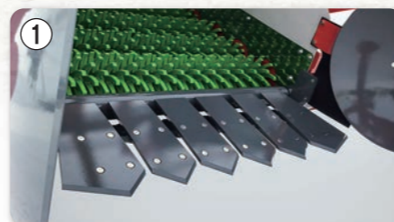
掘取刃は6ポイントショベル型で、掘取りの抵抗を少なくすると同時に、石礫が挟まりにくい形状になっております。
